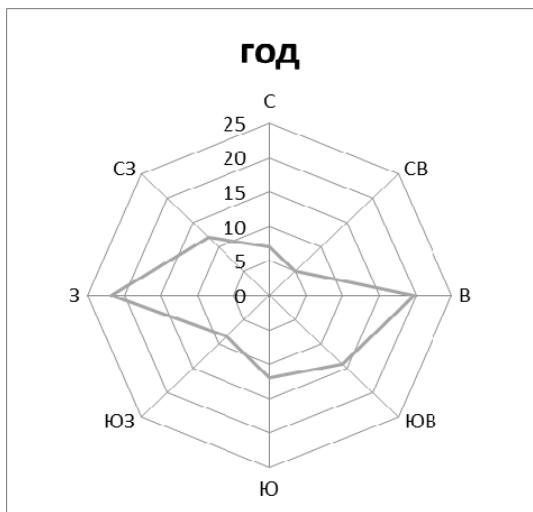
Рисунок 2.1 Роза ветров за год
